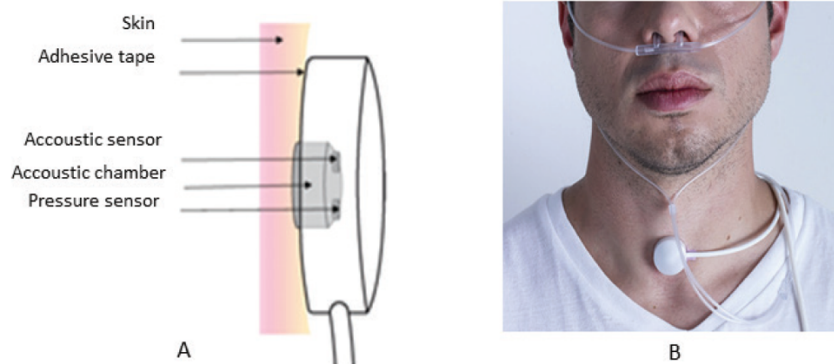
Figure 6 - Capteur associant un capteur acoustique et un capteur de pression (A). Méthode de fixation du capteur au-dessus de la fourchette sternale (B).
